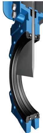
ZWISCHENSTELLUNG
